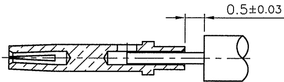
CONTACT PIN ASSEMBLY (中心針組裝)
